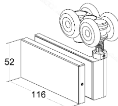
HR610-1 Roller Hinge
