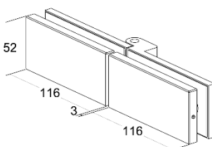
HN610-2 Hinge
